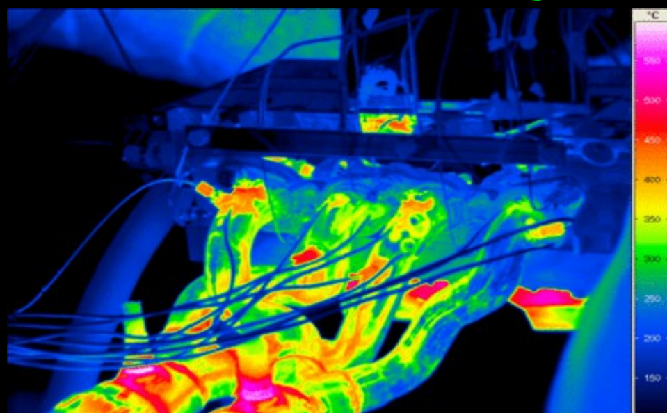
Výfukové svody
