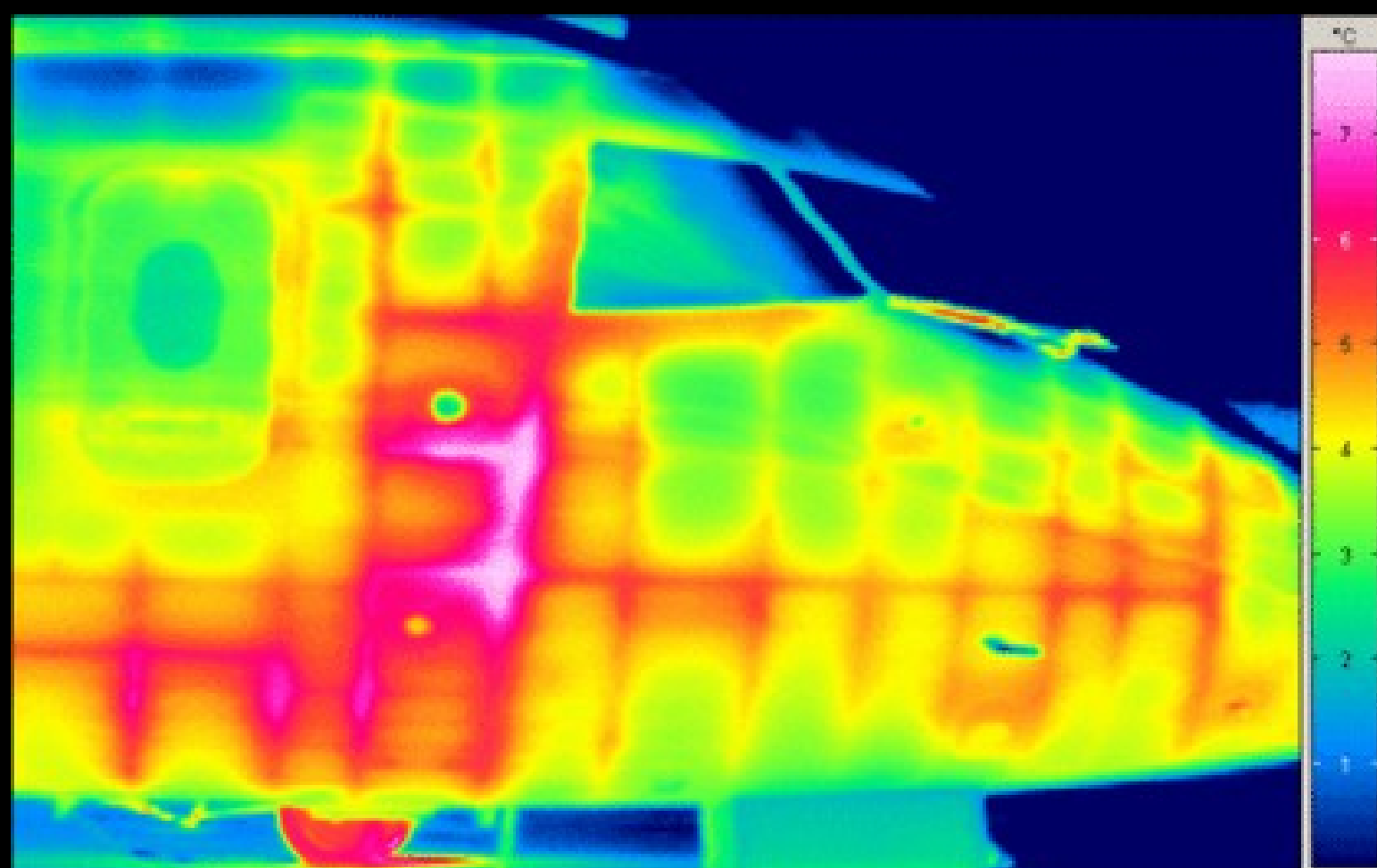
Kontrola trupů
