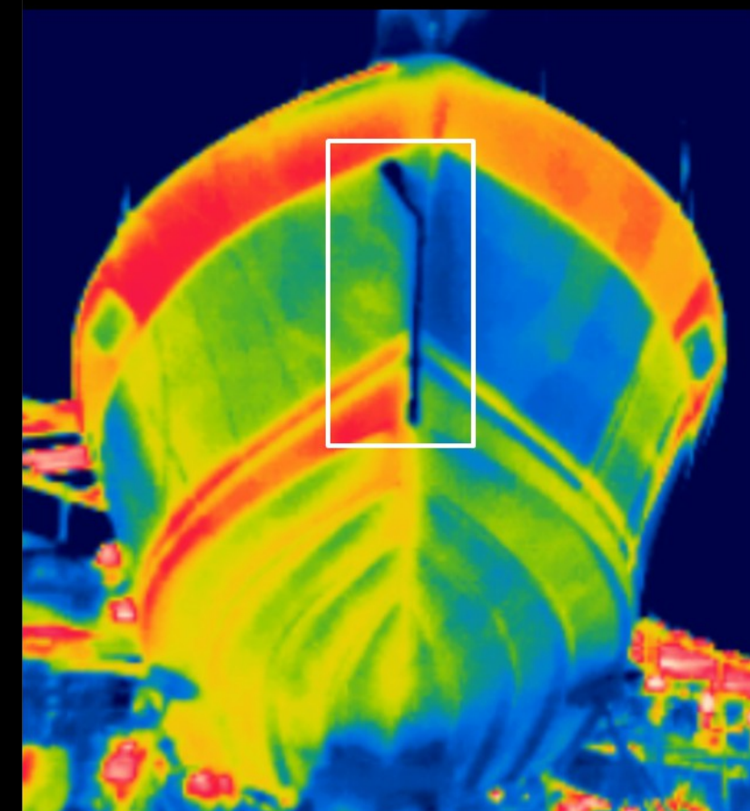
Trhliny trupů lodí Moisture Detection
