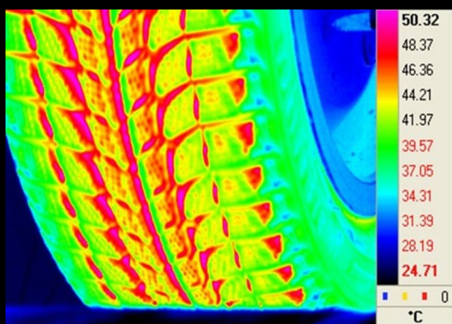
Sjíždění pneumatik
